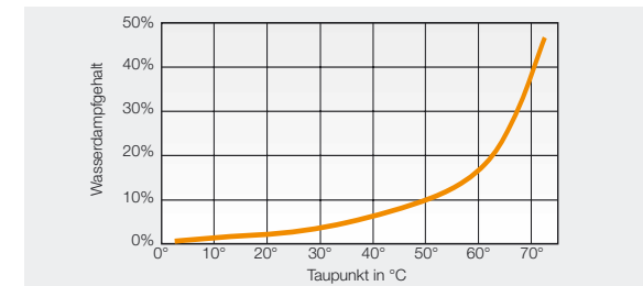
Abb. 11: Wasserdampfgehalt in Abhängigkeit vom Taupunkt (Luftdruck: 1013 mbar)
