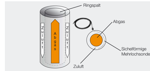
Abb 26: O 2 -Ringspaltmessung mit sichelförmiger Mehrlochsonde
