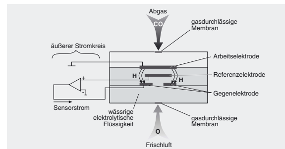
Abb. 34: Schemadarstellung eines Kohlenmonoxid-Sensors
