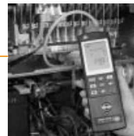
67 Gasdruckprüfung mit testo 312-1/2
